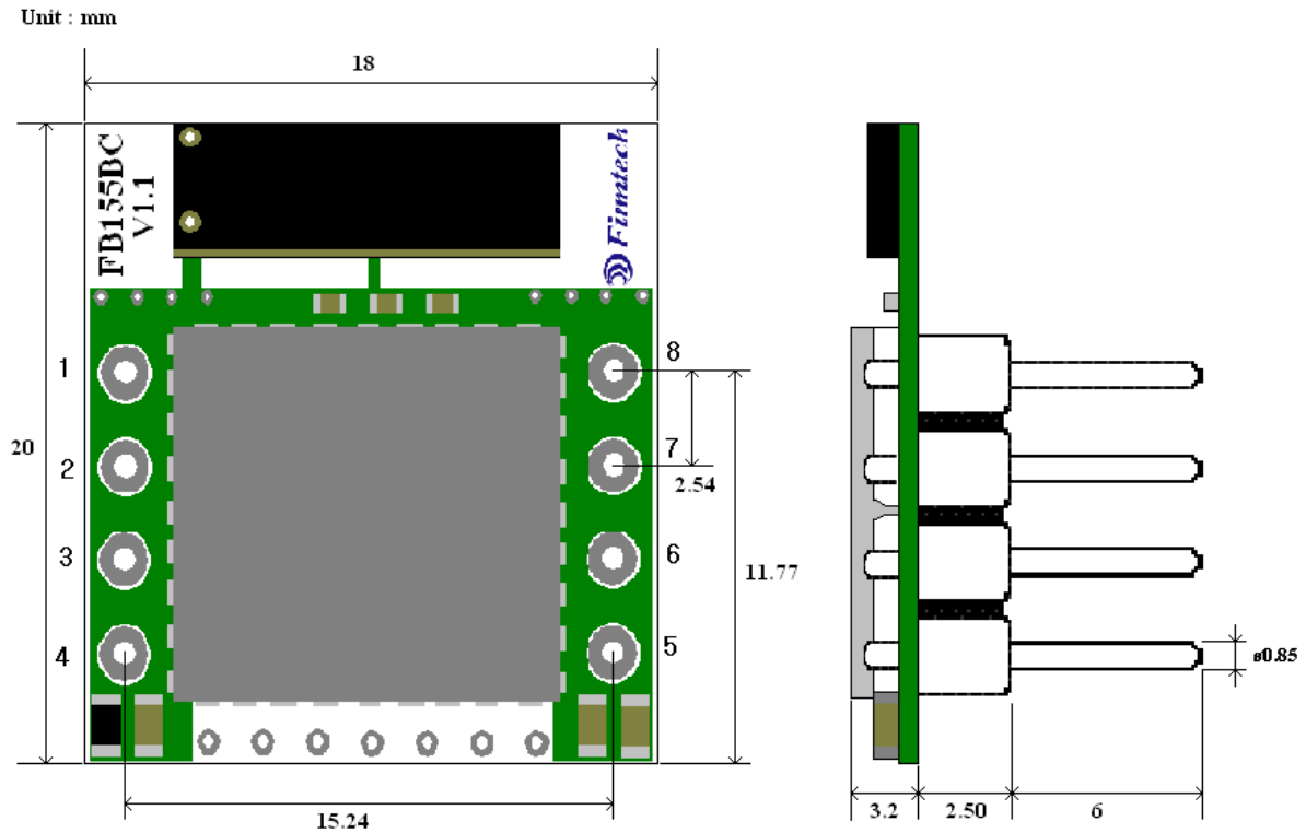
<그림 4-1 FB155BC Dimension>
